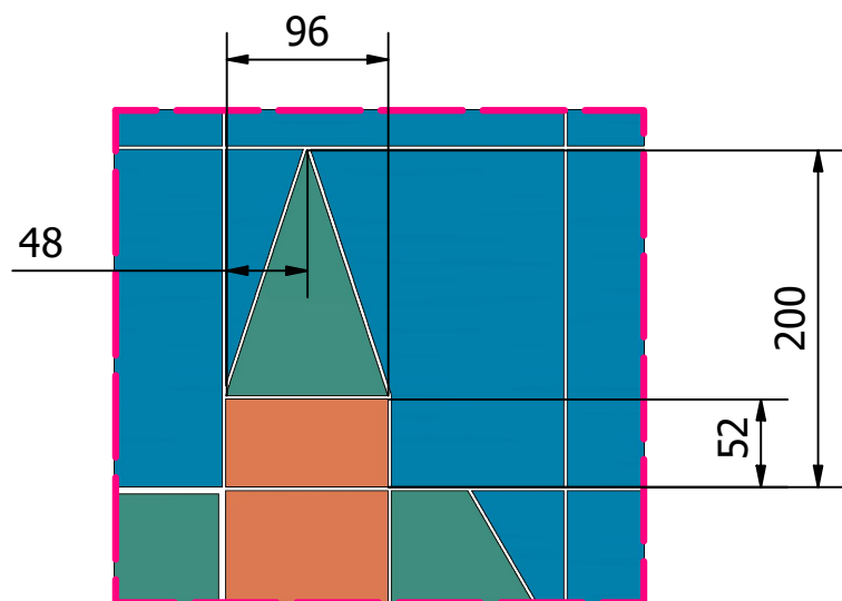
D03 DETALJER LITET TORN ( 1 : 5 )
