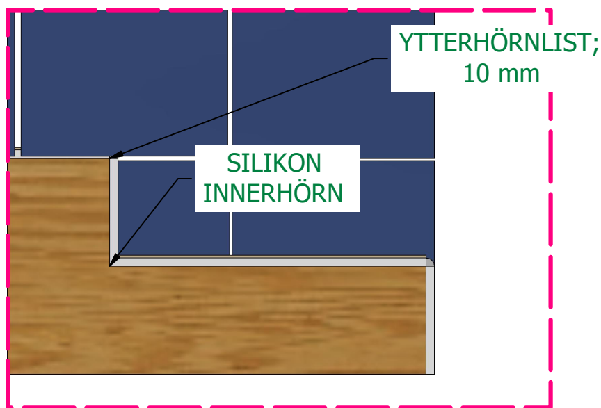
D01 DETALJER INNER- OCH YTTERRHÖRN ( 1 : 5 )
