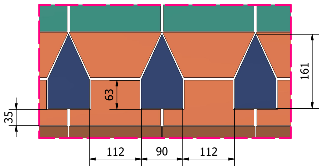
D04 DETALJER FÖNSTER ( 1 : 5 )
