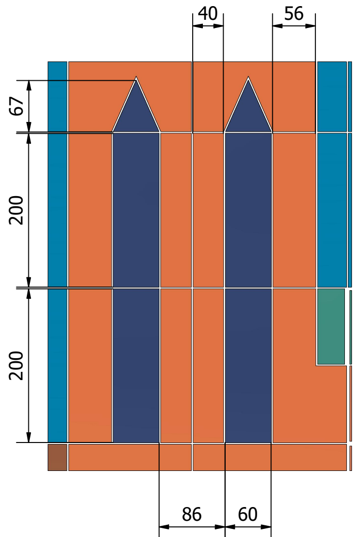
D005 DETALJER FÖNSTER ( 1 : 5 )
