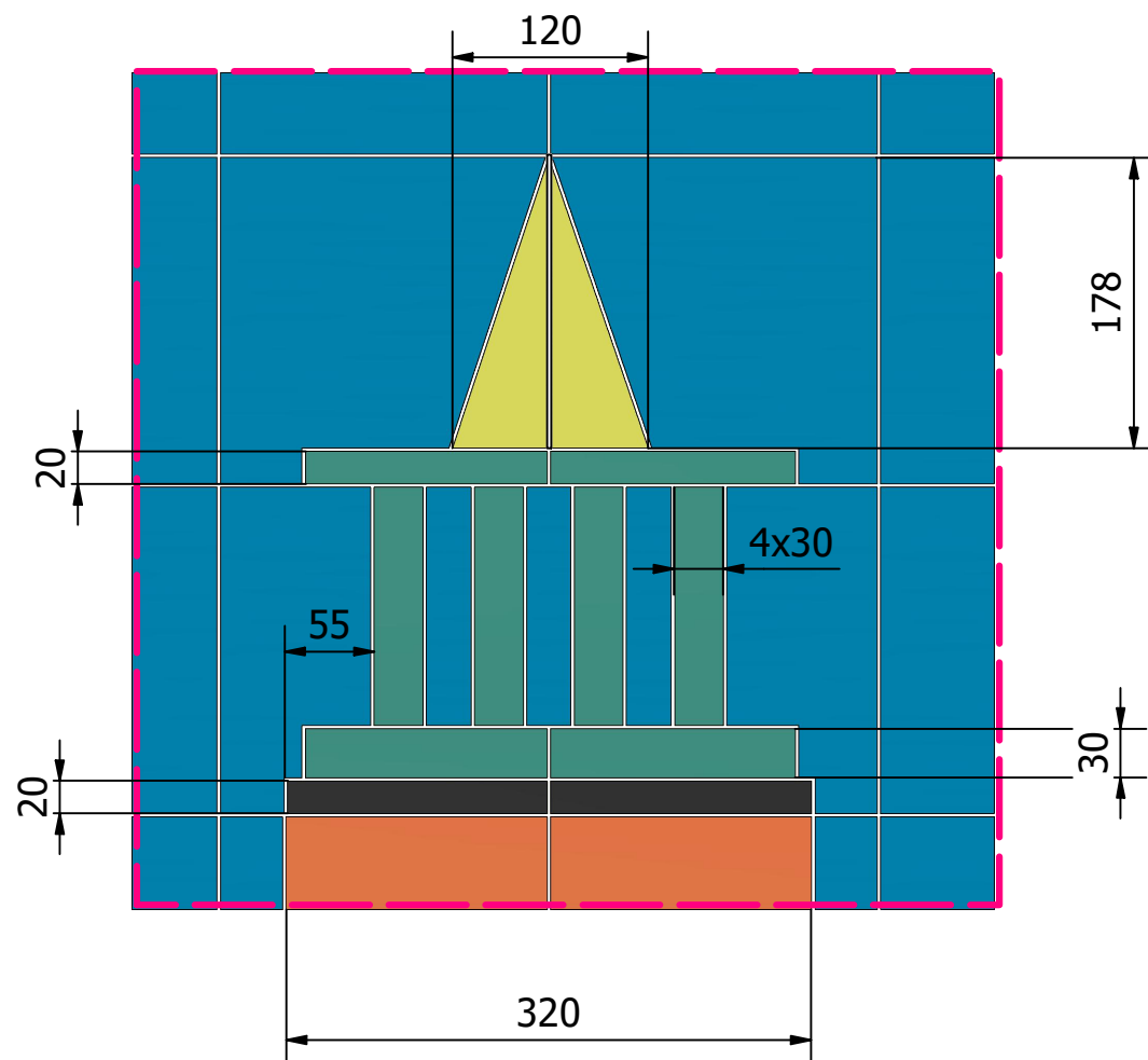
D02 DETALJER KLOCKTORNET ( 1 : 5 )
